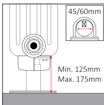
PGT 60 per pavimento finito
