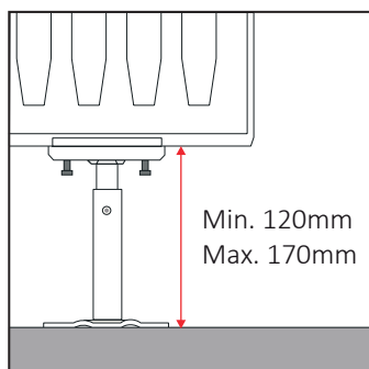
PX3 für Fertigbode
