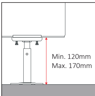
PX3-P für Fertigbode
