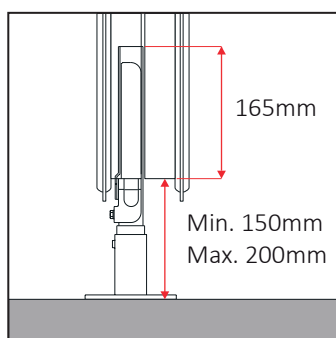
PK3 für Fertigbode
