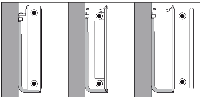
F7L3 10-11 mit Gitter
